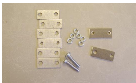
Kabelavlastningsatts
