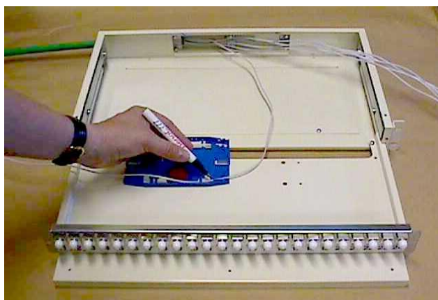
Märkning av tub för skalning.
