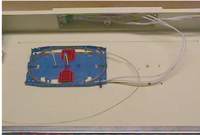
Tuber skalade och fibrer nerslingade i kassetten 1.
