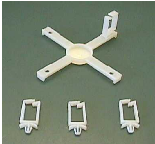
1 OFSB och 4 LWS-A hållare.
