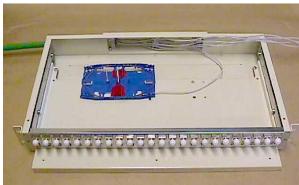
Tub fäst i kassett.
