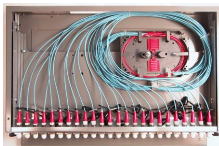
Kopplingspanelen sedd framifrån.
