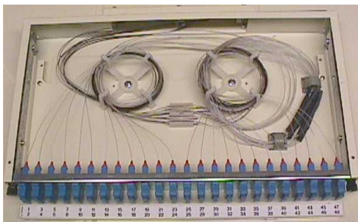
Box med bandfiber skarvat mot fanouter alternativ 1.
